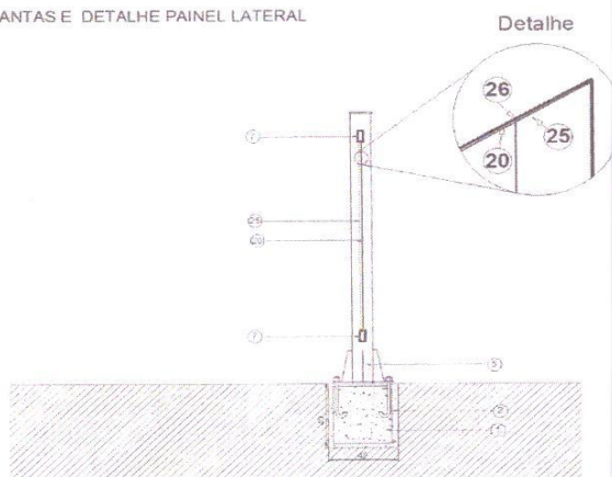
Detalhamento - Painel Lateral Módulo 1,82m x 3,00 m
