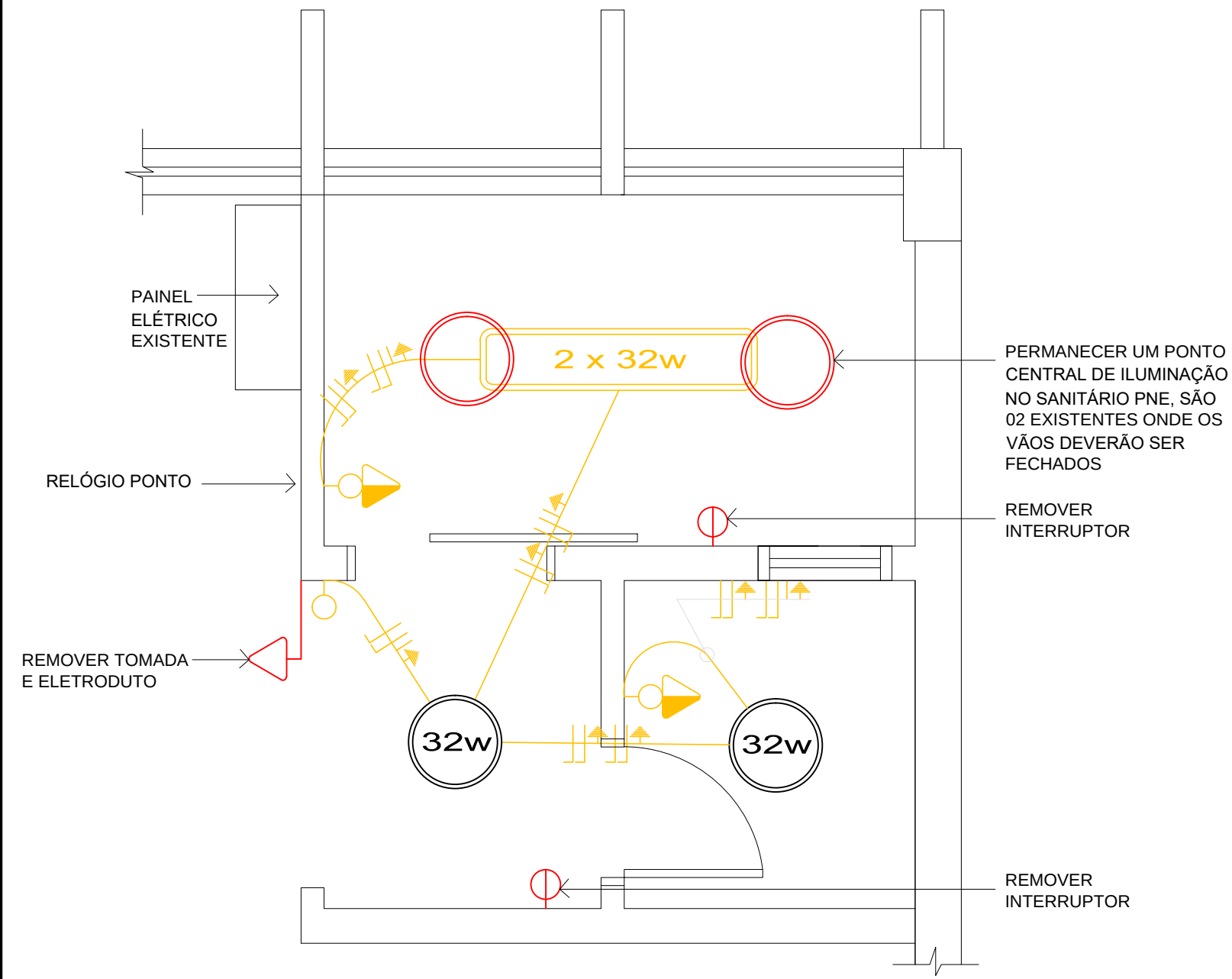
PLANTA BAIXA ELÉTRICO ESC. 1/25
