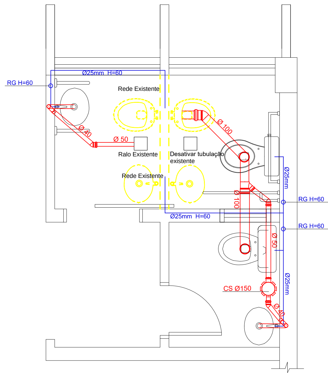
PLANTA BAIXA HIDROSSANITÁRIO ESC. 1/25
