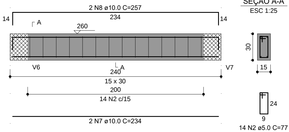
V8 ESC 1:25
