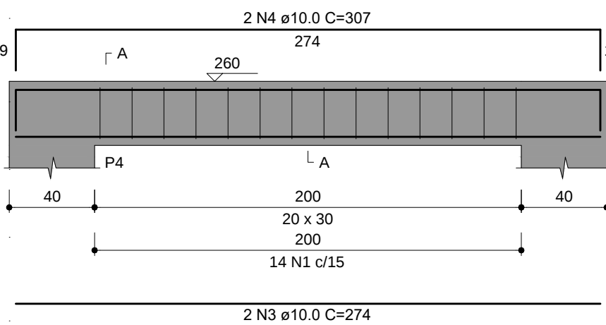
V5 ESC 1:25
