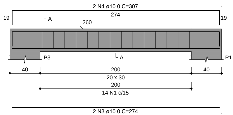
V3 ESC 1:25
