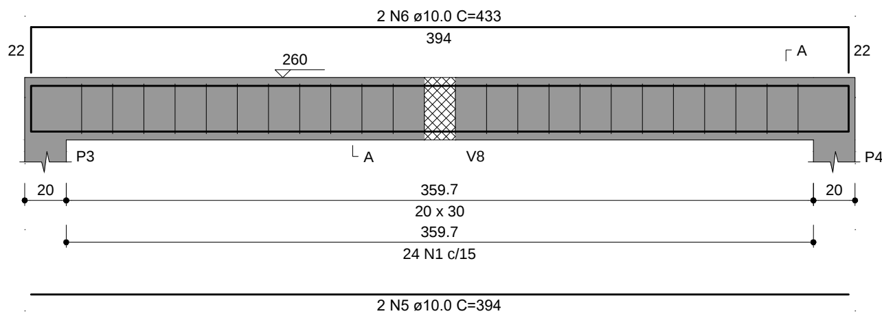
V6 ESC 1:25
