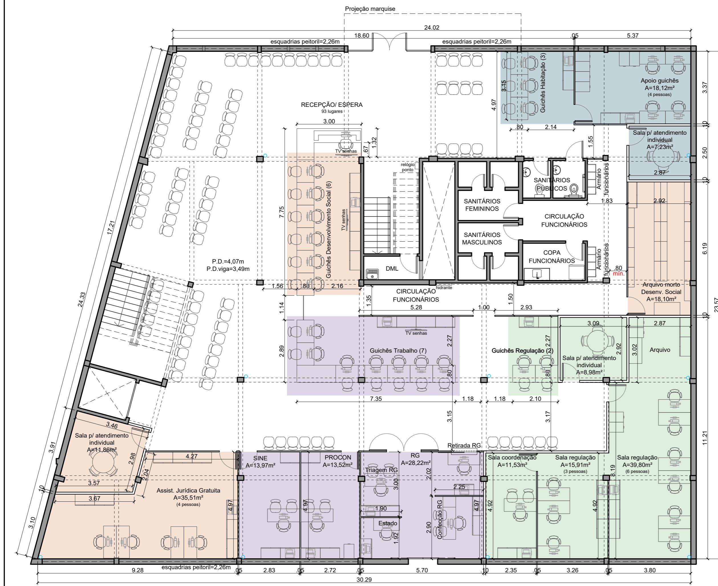
PLANTA BAIXA - PAVTO. TÉRREO Esc. 1/100
