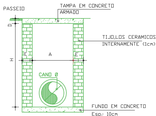
CORTE TRANSVERSAL
