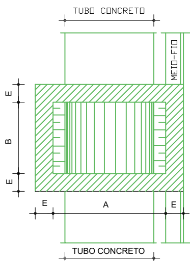
PLANTA BAIXA
