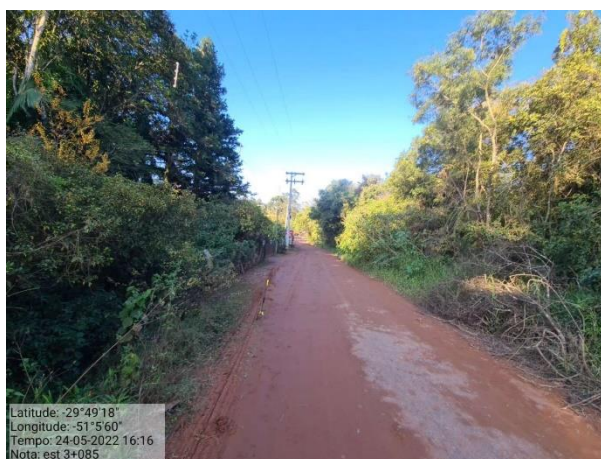
Foto 16: Vista geral do trecho - Estaca 3+085m
