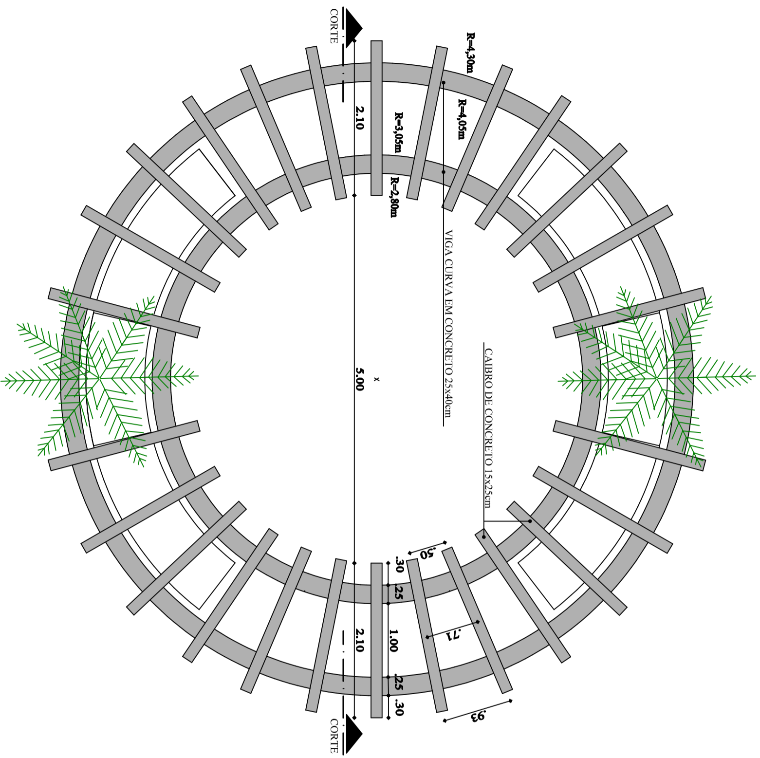
PLANTA BAIXA PERGOLADO - VISTA DE CIMA
