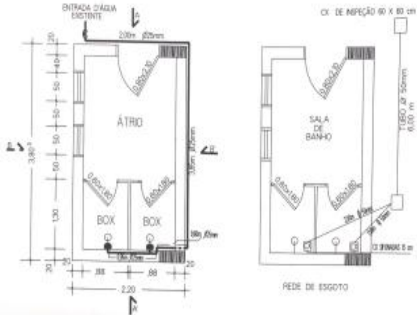
PLANTA BAIXA - SALA DE BANHO CEMITÉRIO PIO XII ESC : 1/50
