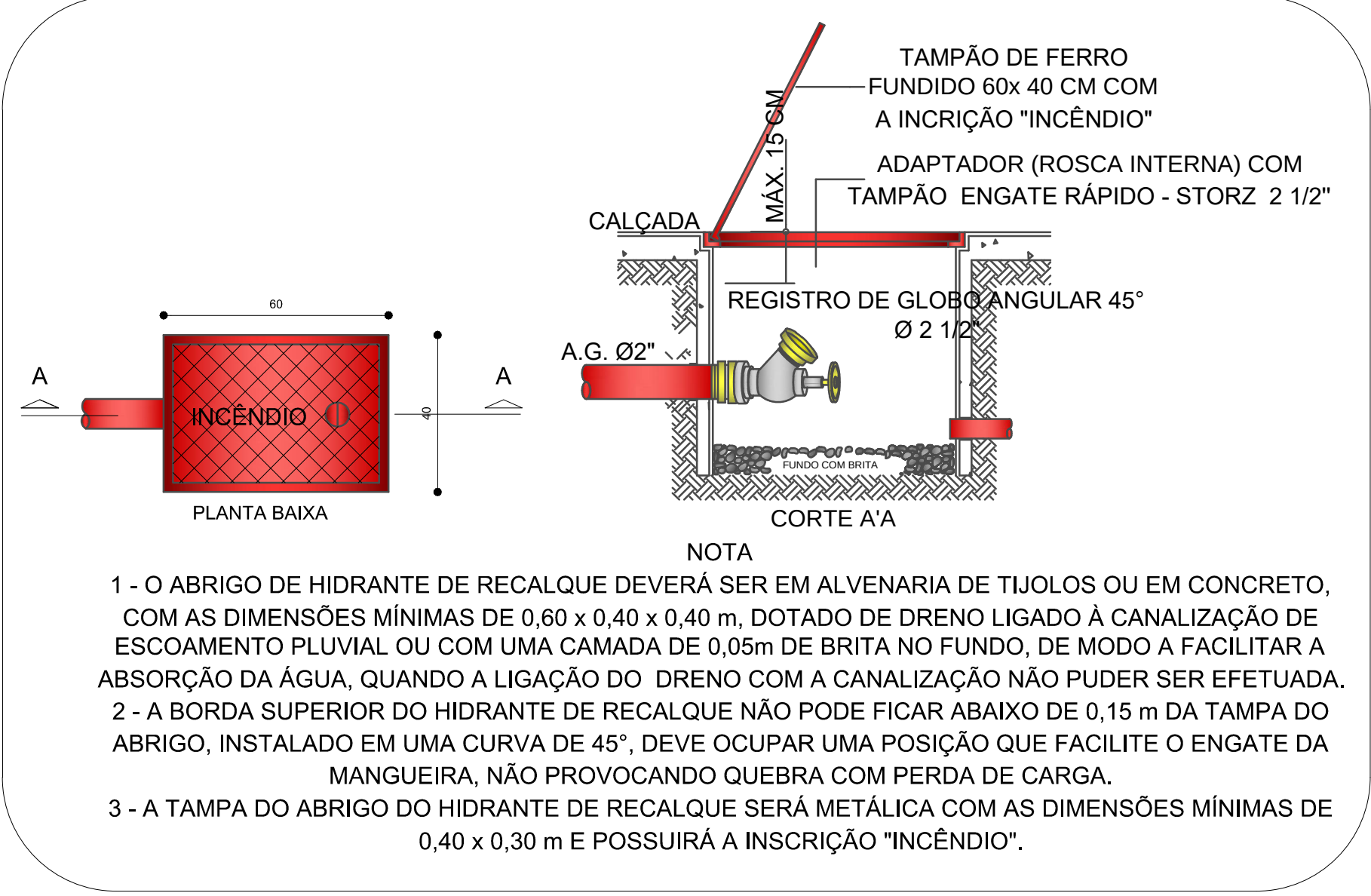
DETALHE 07 - REGISTRO DE RECALQUE
