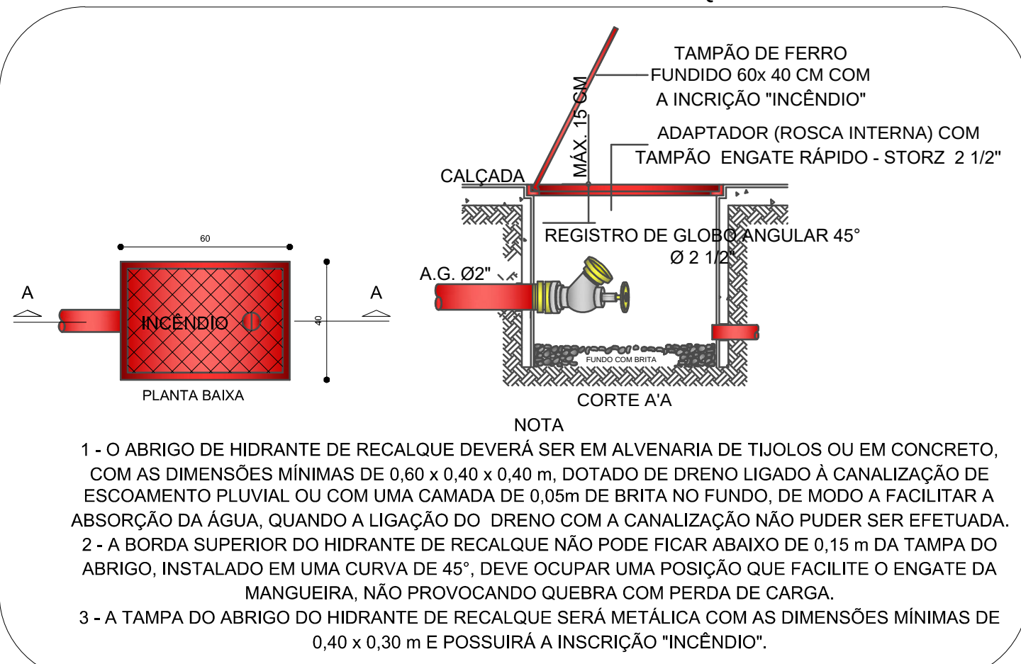
DETALHE 07 - REGISTRO DE RECALQUE
