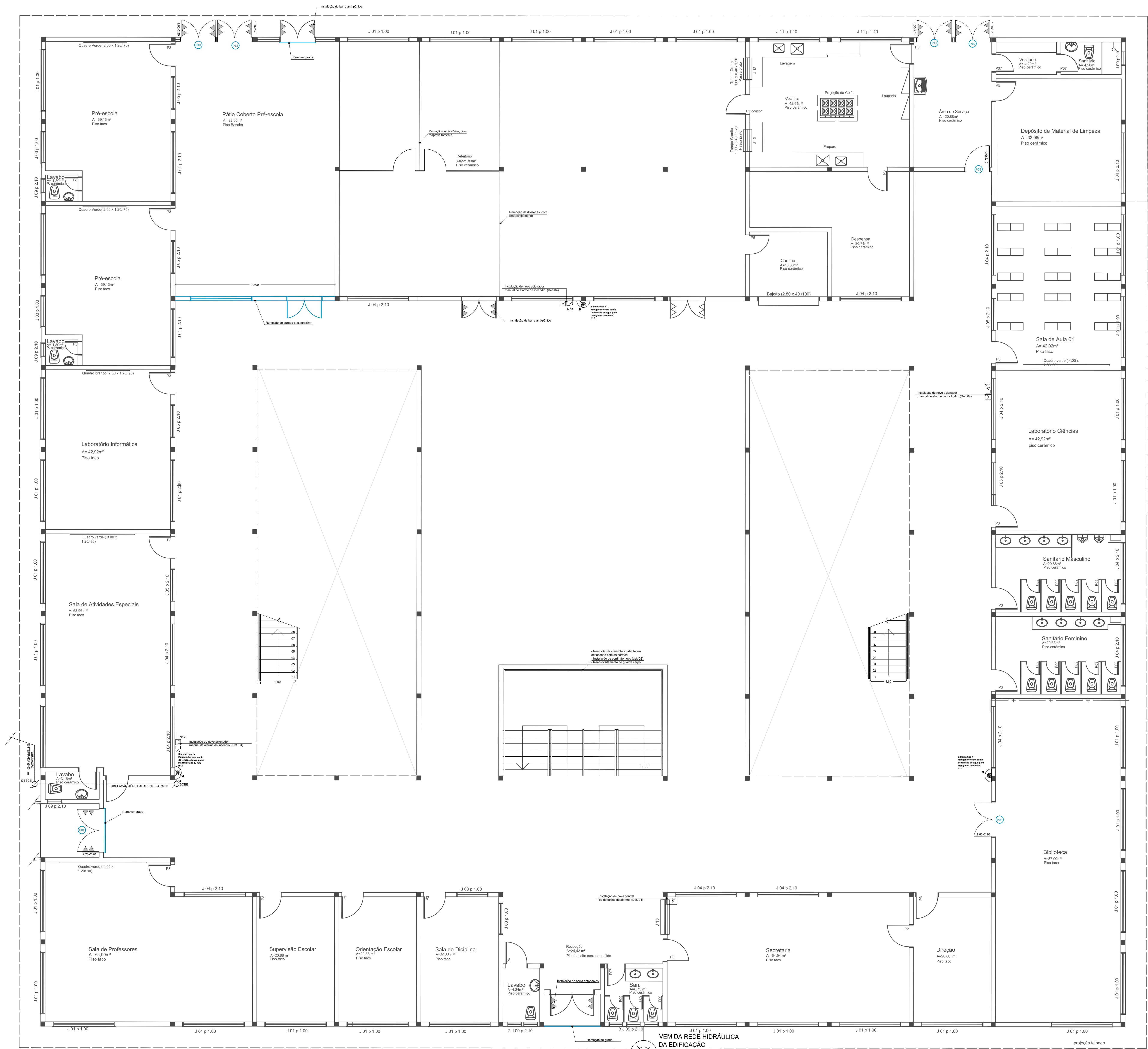
PRÉDIO 1 PLANTA BAIXA PAVIMENTO TÉRREO A=1973,80m²
