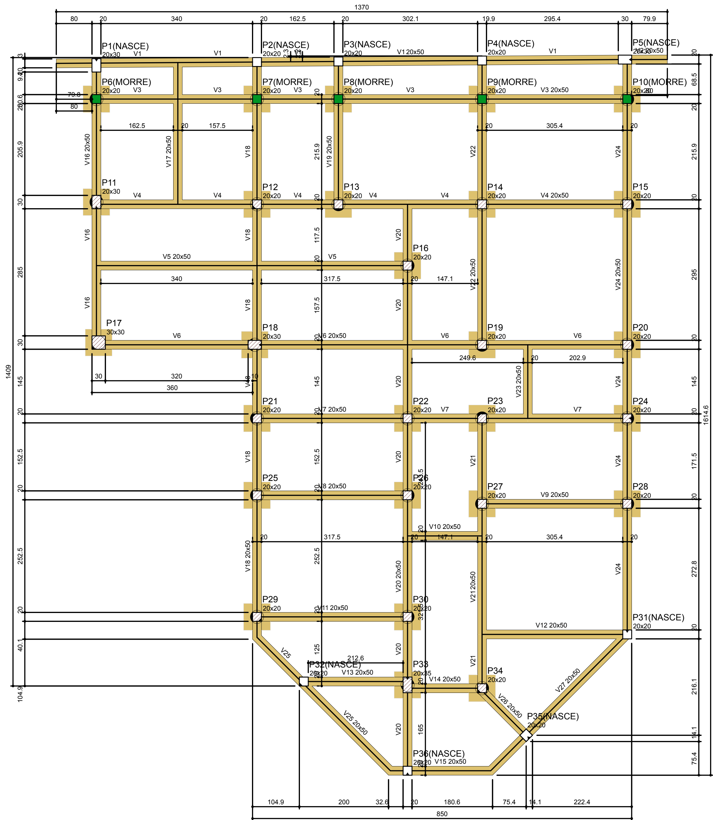
Forma do Pavimento Baldrame escala 1:50
