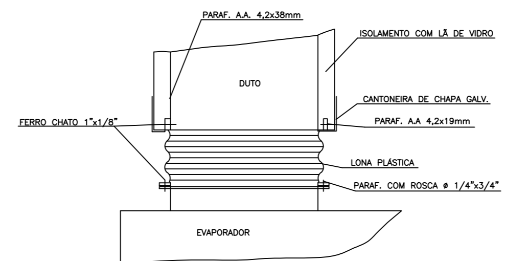
DETALHE CONEXÃO EQUIPAMENTO ESC. SEM
