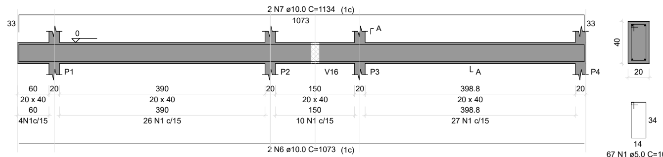
V4 ESC 1:50
