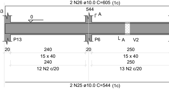
V21 ESC 1:50
