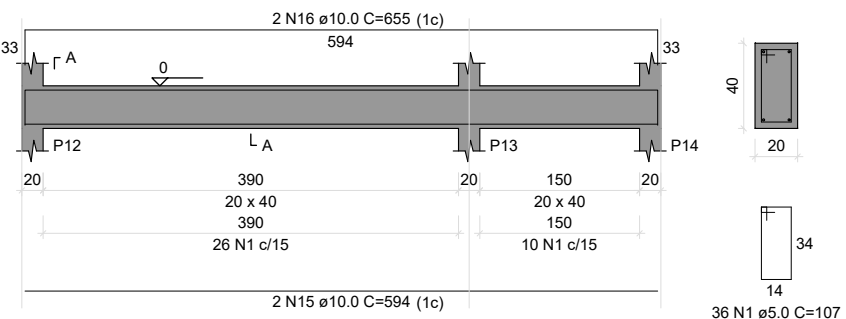
V6 ESC 1:50
