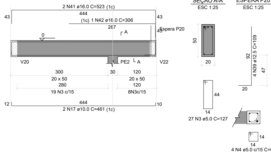
V13 ESC 1:50
