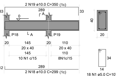
V8 ESC 1:50
