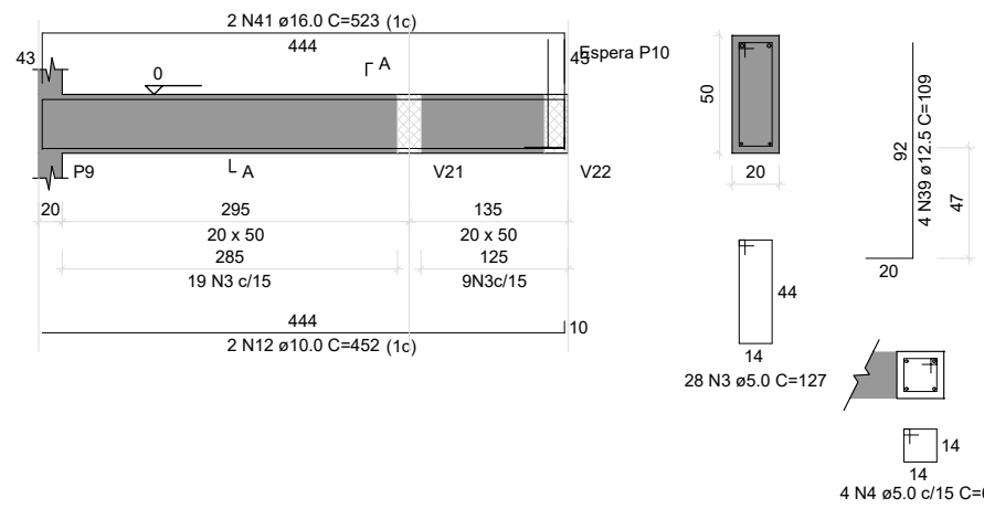
V4 ESC 1:50
