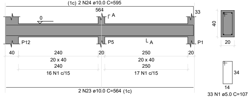
V20 ESC 1:50
