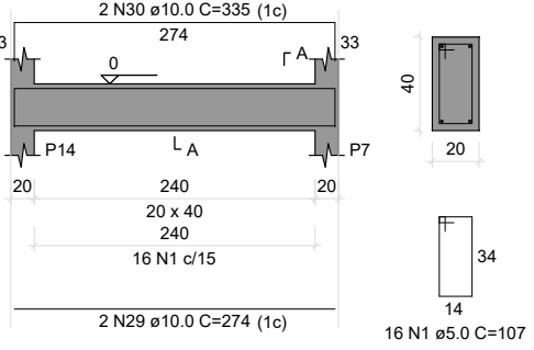
V17 ESC 1:50
