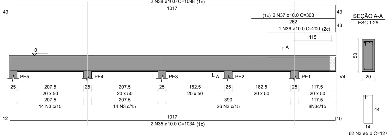
V21 ESC 1:50
