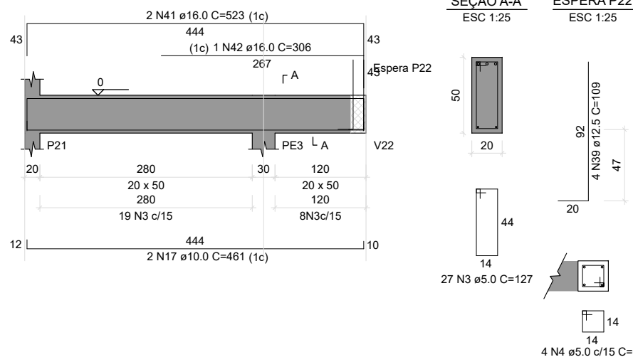
V15 ESC 1:50
