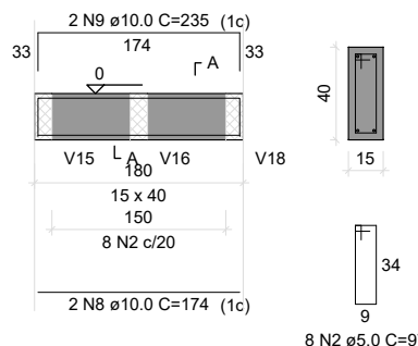
V6 ESC 1:50
