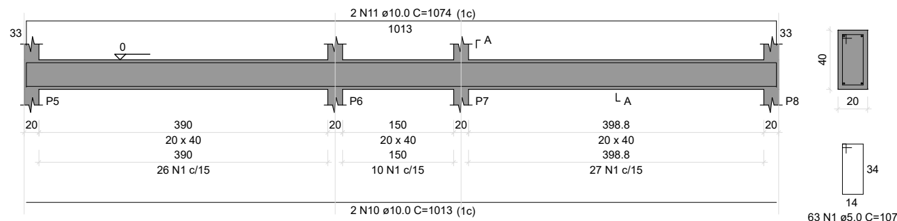
V7 ESC 1:50
