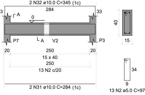
V18 ESC 1:50
