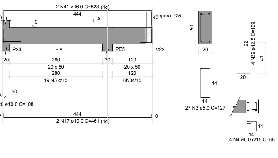
V18 ESC 1:50
