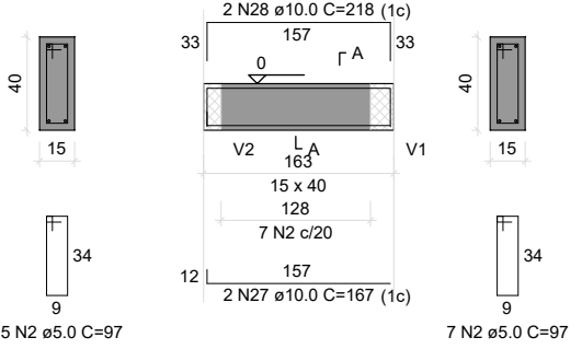
V16 ESC 1:50
