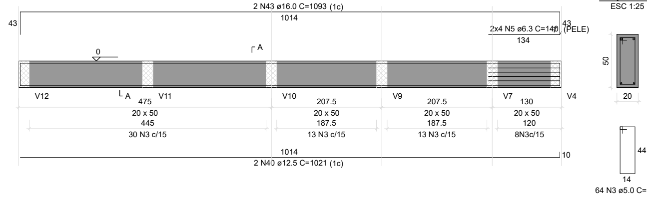
V22 ESC 1:50
