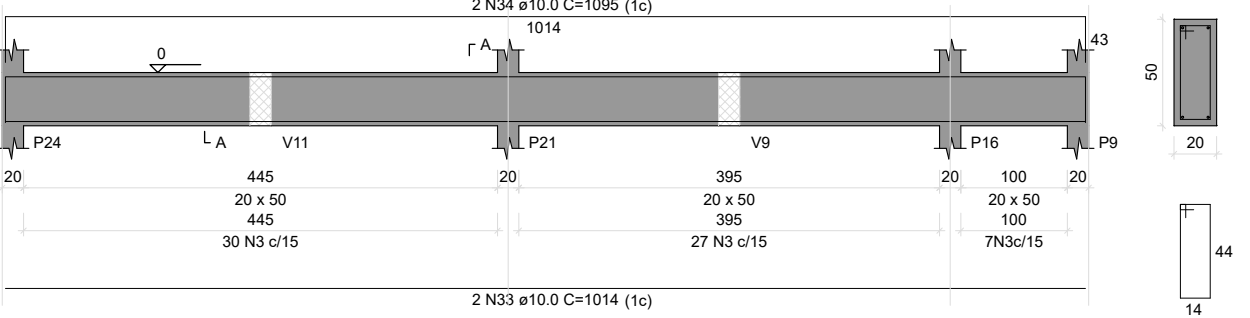
V20 ESC 1:50
