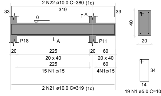
V19 ESC 1:50
