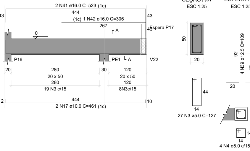
V12 ESC 1:50
