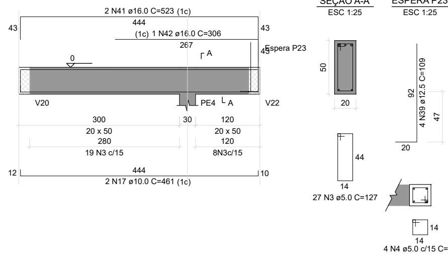
V16 ESC 1:50
