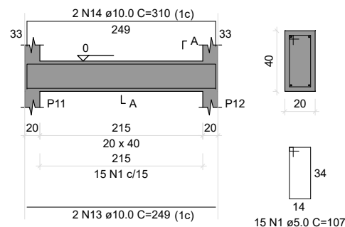
V5 ESC 1:50
