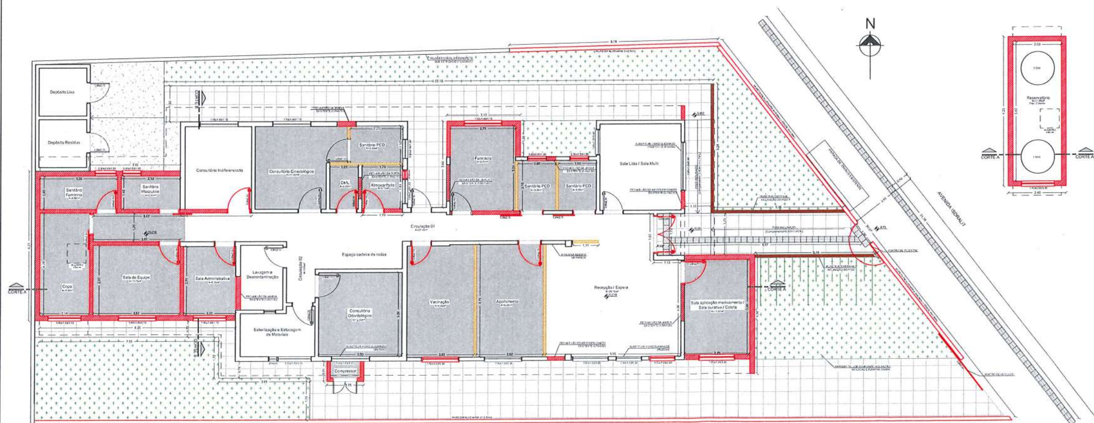
PLANTA BAIXA - OBRA ESC. 1/75
