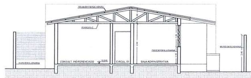
CORTE BB ESC. 1/75
